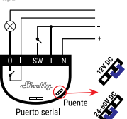
fig.2 Fuente de Alimentación: 12V; 24-60 DC
