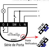
fig.2 Fonte de energia: 12V; 24-60V DC
